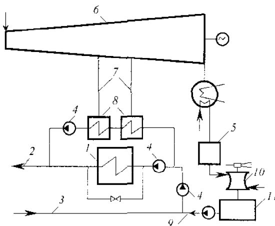
Рис. 5. Схема ТЭЦ с параллельным включением пиковых водогрейных котлов и основных сетевых подогревателей: 1 - пиковый водогрейный котел; 2, 3 - подающий и обратный трубопроводы теплосети; 4 - сетевой насос; 5 - узел умягчения; 6 - теплофикационная турбина; 7 - отопительные отборы пара; 8 - сетевые подогреватели; 9 - трубопровод подпиточной воды; 10 - вакуумный деаэратор; 11 - бак-аккумулятор
